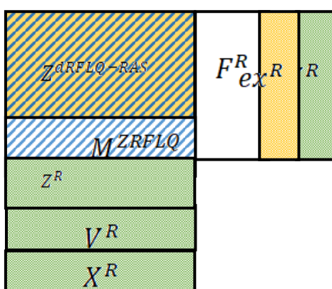
الف) جدول RIOT به روش FLQ با بردار پسماند ارزش افزوده
