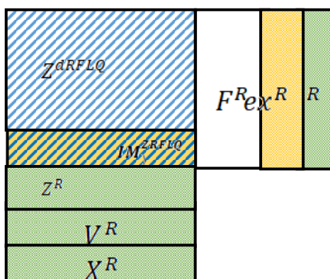
ج) جدول RIOT به روش جدید FLQ با بردار آماری ارزش افزوده
